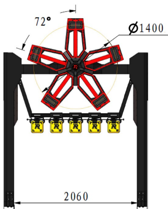
图 4-12 能量机关示意图
