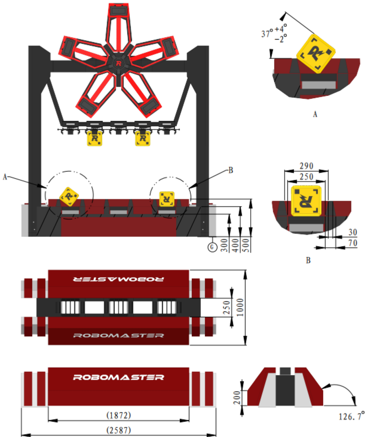
图 4-3 资源岛尺寸示意图
